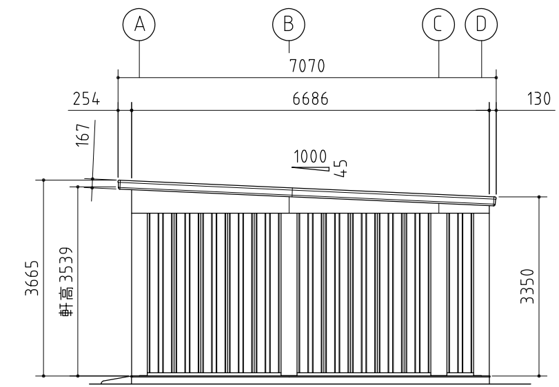
側面図
