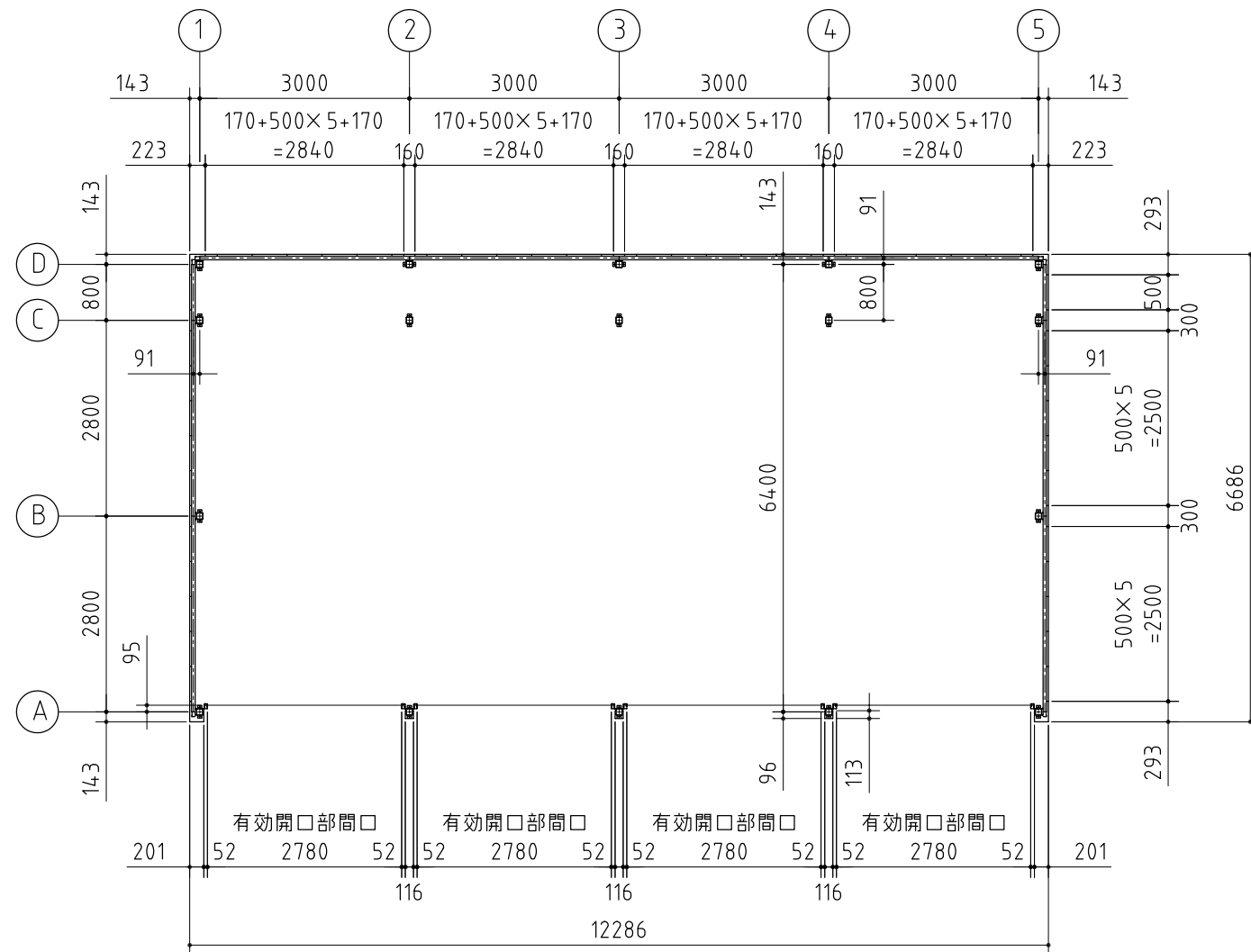
平面図
