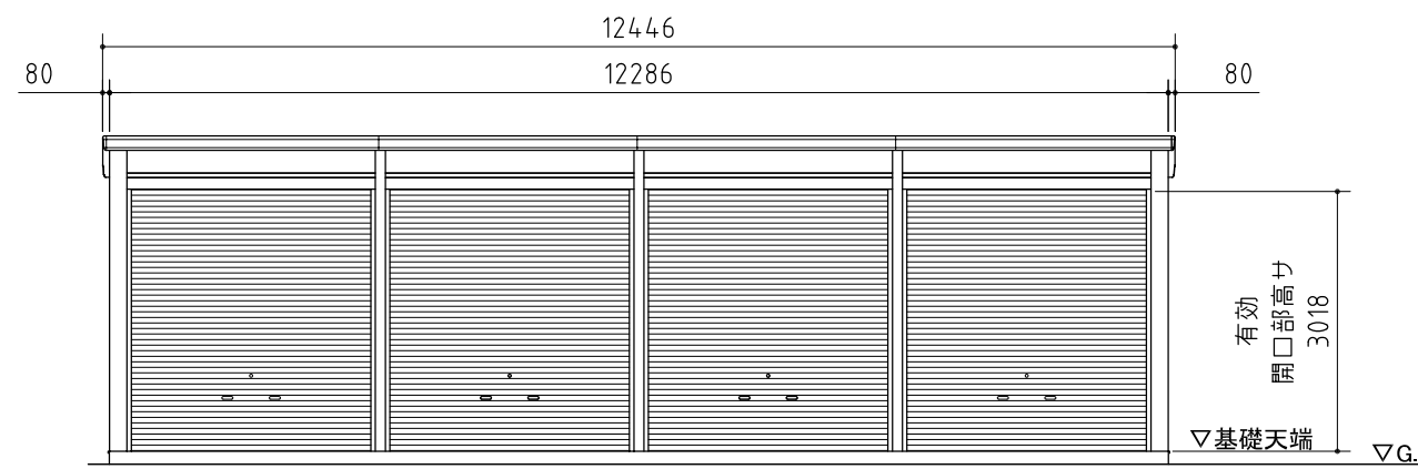
正面図
